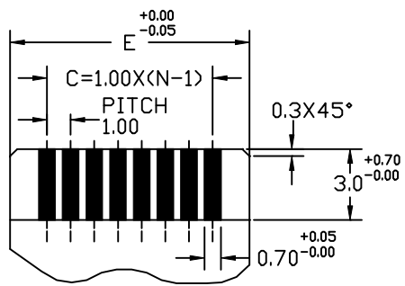
FLEXPRINT CABLE REFERENCE DIM.
